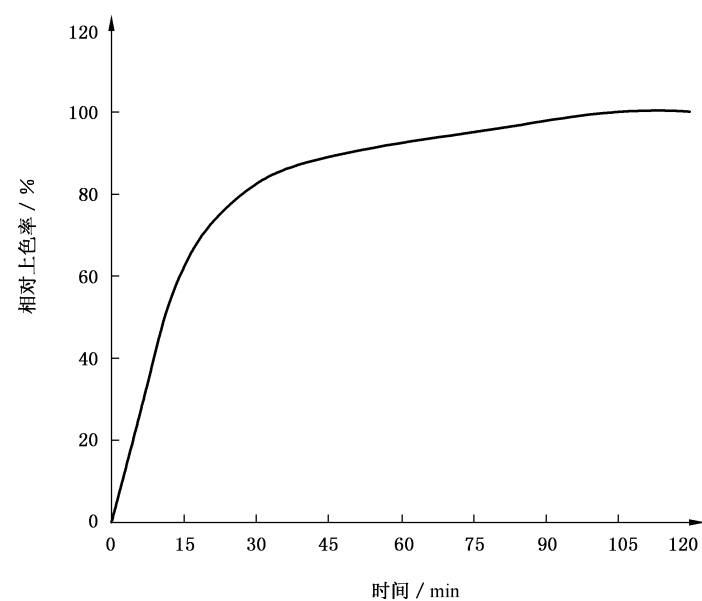
图 A.1 硫化黄棕 6G 150% 上染速率曲线
